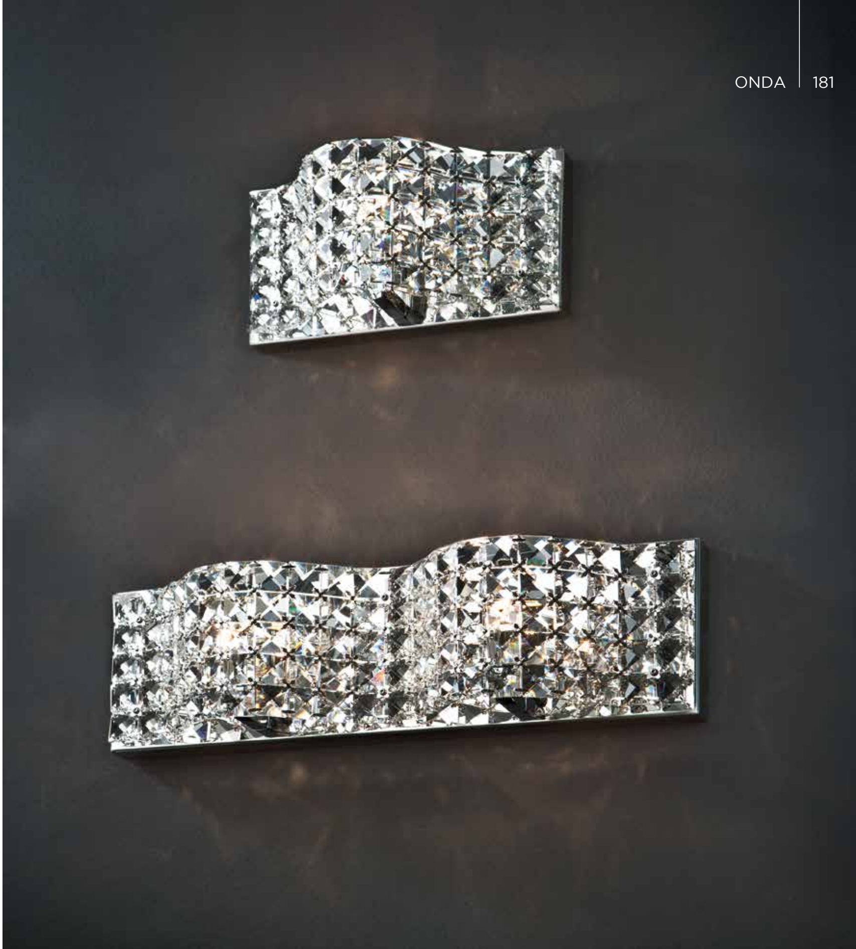
△ 160320 (pequeño/small) ppuntos/points 160 ↔ 25 ↑13 ↘ 8 cm 1 G9 LED 6W 550 lumen / 3.000 K Peso/weight 0,8 Kg Medidas del florón ↔ 25 ↑13 ↘ 2 cm Sizes of the canopy
