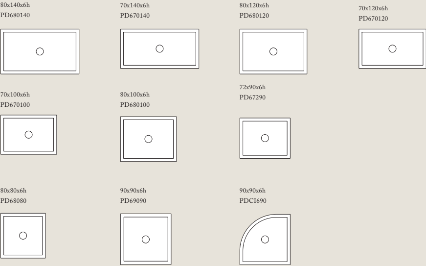
installazione da appoggio floor installation
